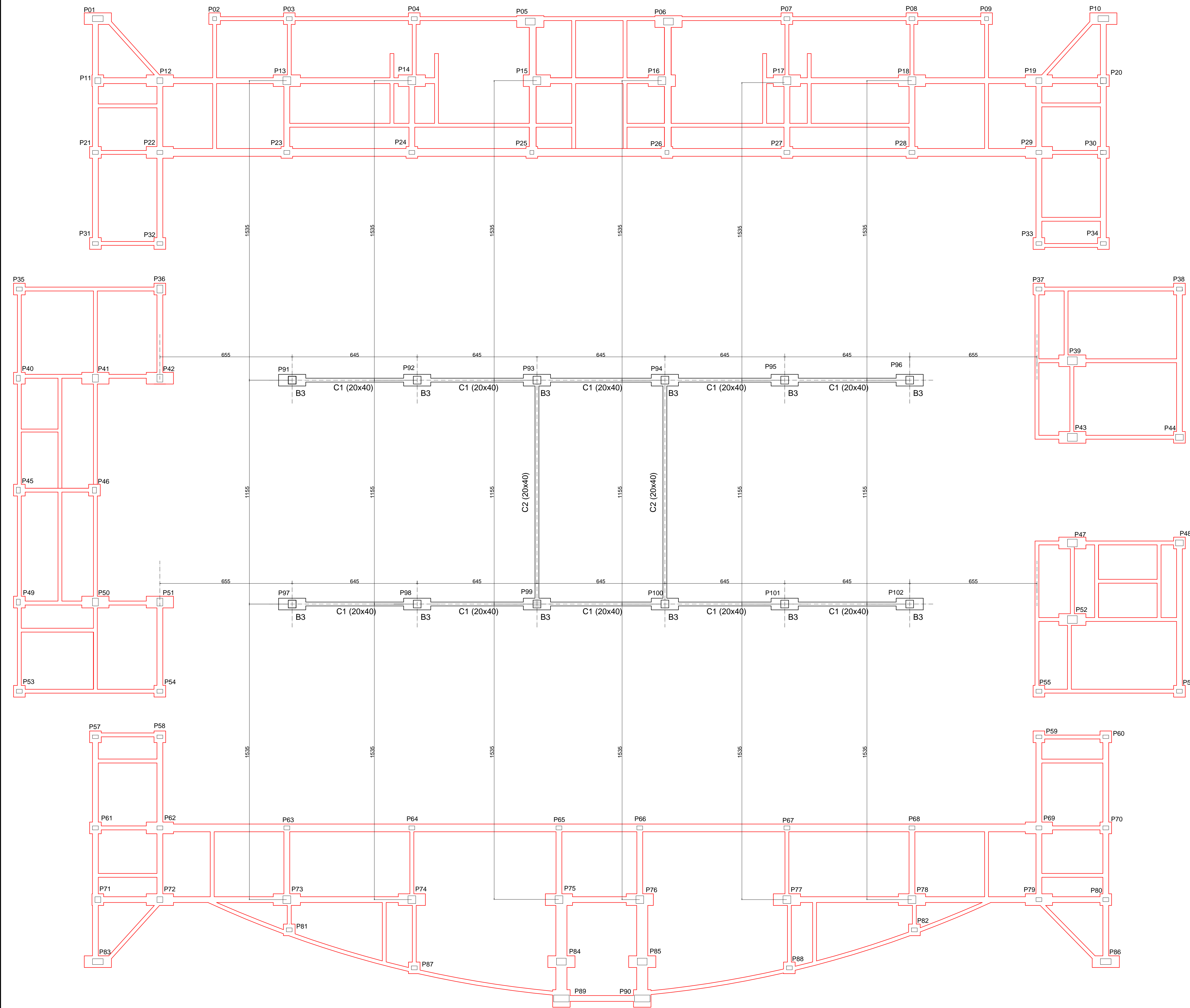
1 PLANTA DE FUNDAÇÕES LOCAÇÃO DE PILARES, CINTAS E BLOCOS ESC: 1/100
