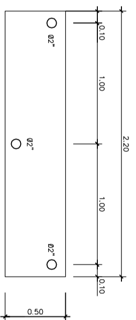
LOCAÇÃO DOS MASTROS PLANTA – ESC.: 1 : 25
