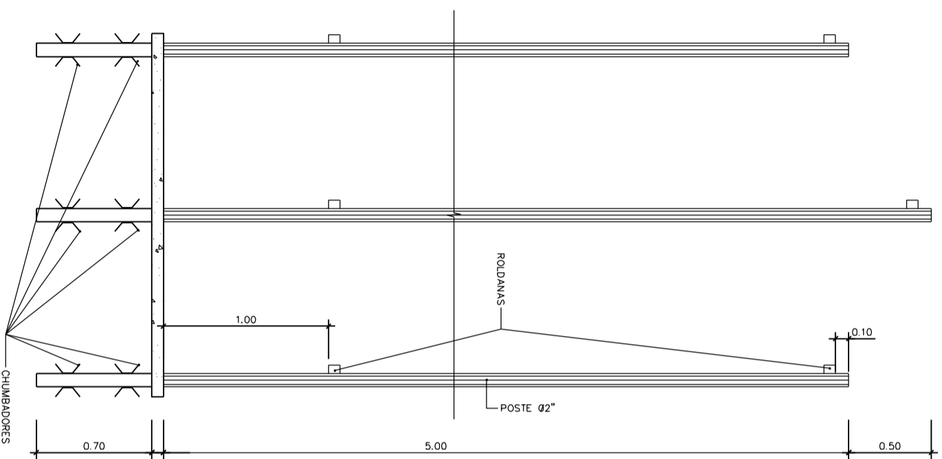
MASTROS DE BANDEIRAS DET. VISTA – ESC.: 1 : 25
