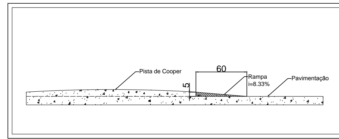
VISTA LATERAL DA RAMPA DE COMPENSAÇÃO ENTRE A PISTA DE COOPER E A PAVIMENTAÇÃO Escala: 1/25
